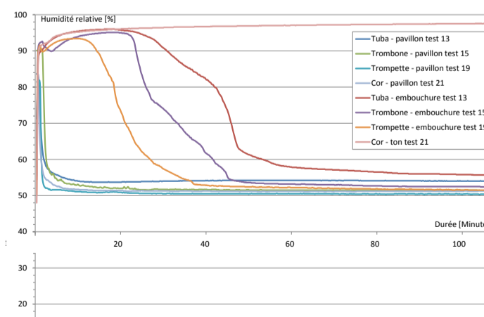
Die relative Feuchtigkeit der Luft in Instrumenten, die mit dem Ventilator getrocknet werden, entspricht ausser bei den Hornbögen (hellrot) nach kurzer Zeit derjenigen der Aussenluft. Verhindert dies Korrosion? (Grafik: E.Cornet)
